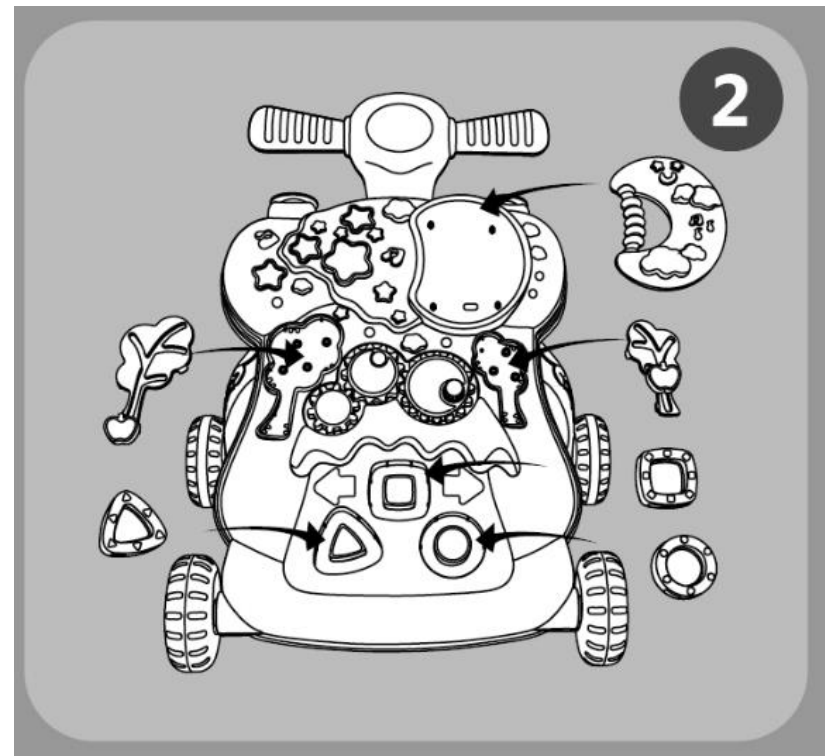
Como se muestra en la figura 2, encastrar los accesorios delanteros.
